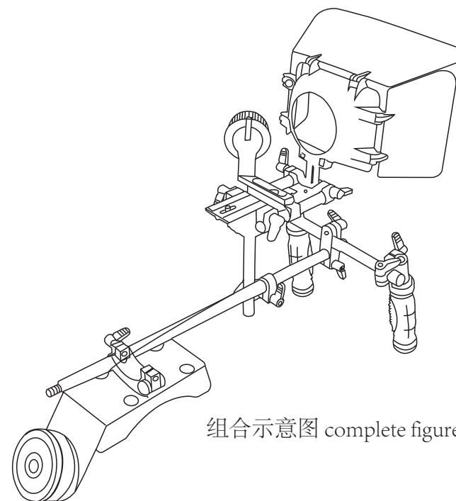
安装分解示意图 installation figure
